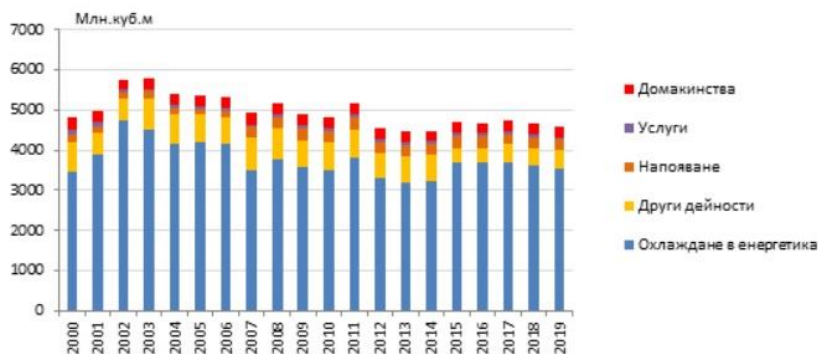
Фигура 2.1.3-1. Използвана вода по основни икономически сектори общо за страната; Източник: ИАОС, Национален доклад за състоянието и опазването на околната среда, 2020 г.
