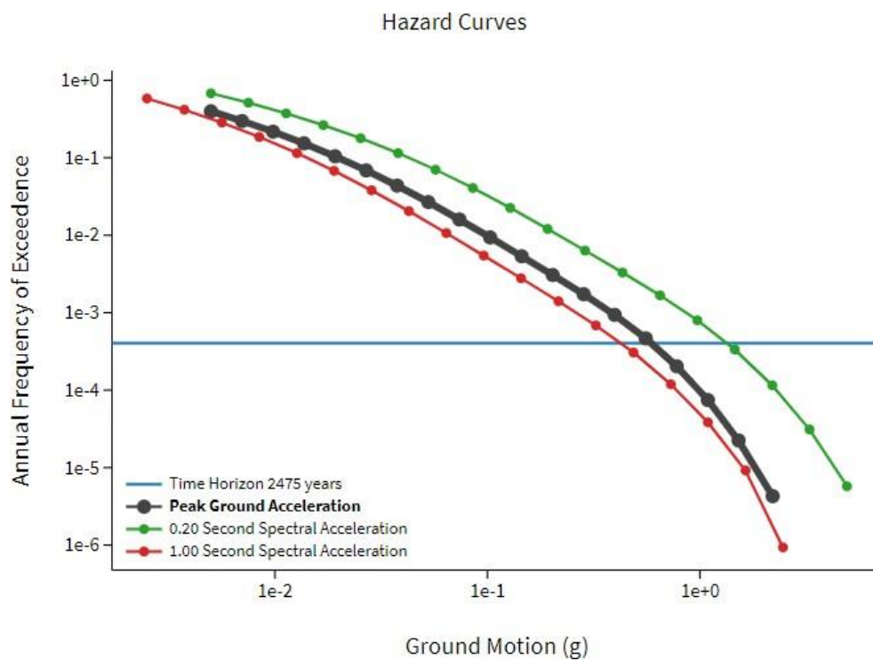
Фигура 3. Пример за крива на опасността от земетресение, която показва вероятността от превишаване на върховото ускорение на земята на дадено местоположение.
