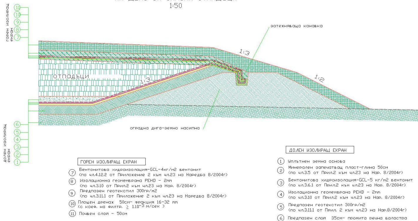
ДЕТАЙЛ-ДОЛЕН И ГОРЕН ИЗОЛИРАЩ ЕКРАН НА ДЕПО ЗА ОПАСНИ ОТПАДЪЦИ 1:50
